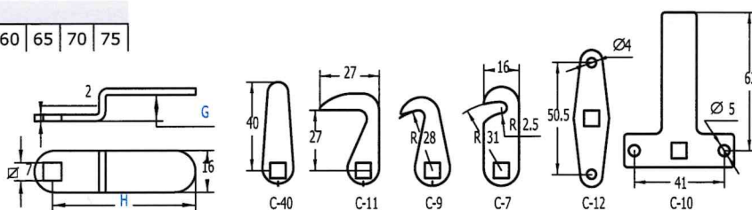
Tirador 0013 Accesorios: página 63.
