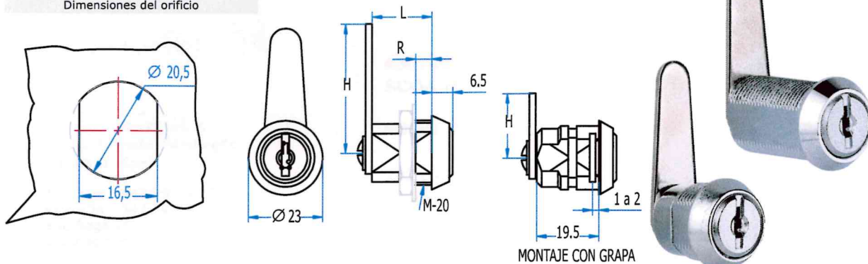
Dimensiones del orificio
