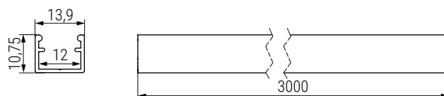
Tapa difusora, para perfil KOY+ Material plástico. Barras de 3 metros.
