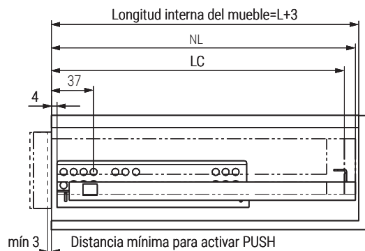
Cajón solapado
