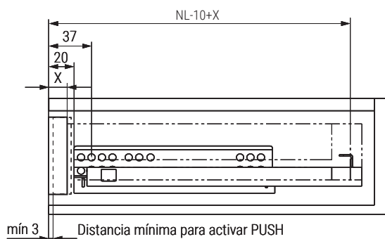
Cajón interno
