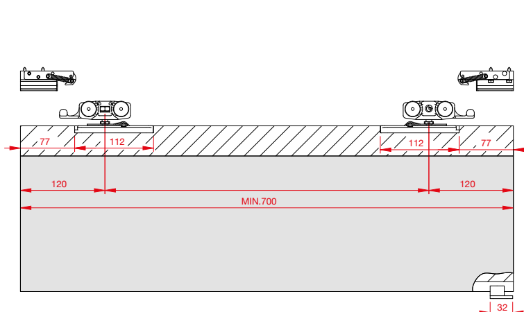
N.2 Hydraulic stopper N.2 Fermi idraulici
