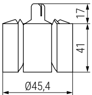
Pieza central con 6 vías para cables
