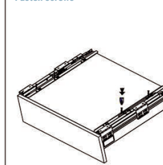
4 Colocación del tornillo rapido/ Fasten screws
