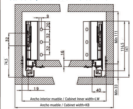
Instalación/Installation Verbox 116mm
