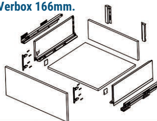
Instalación/Installation Verbox 166mm
