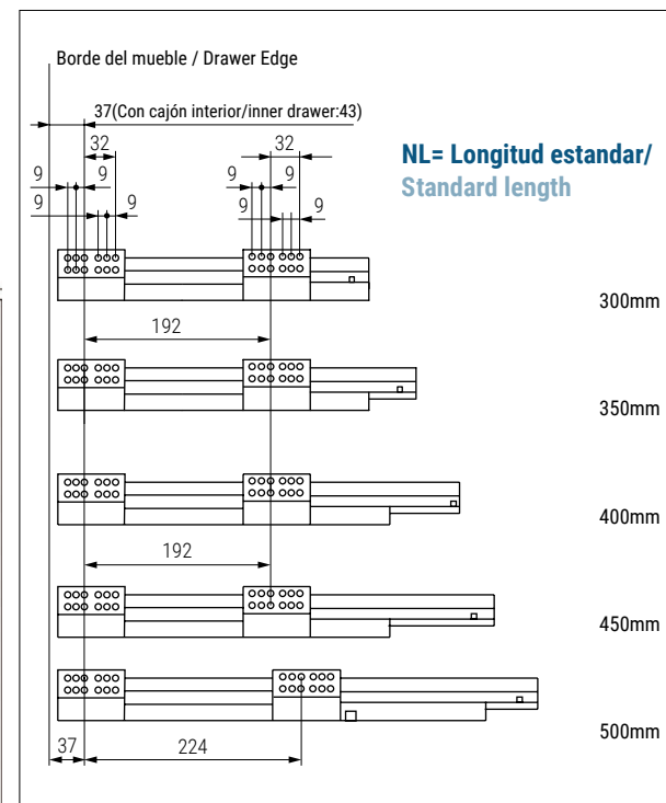
Instalación/Installation Verbox 166mm
