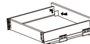
Presiona la tapa y deslízcela dentro el cajón/ Press in cover and slide into the drawer
