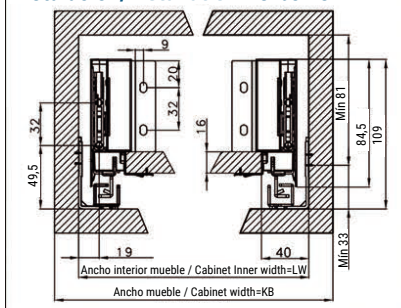
Instalación/Installation Verbox 84mm
