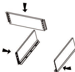
2 Colocación de soportes/ Insert the brackets
