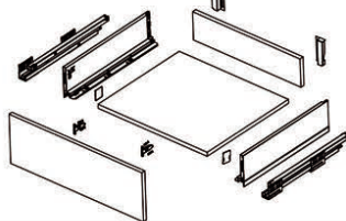
Instalación/Installation Verbox 116mm
