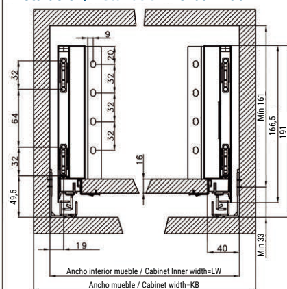
Instalación/Installation Verbox 166mm
