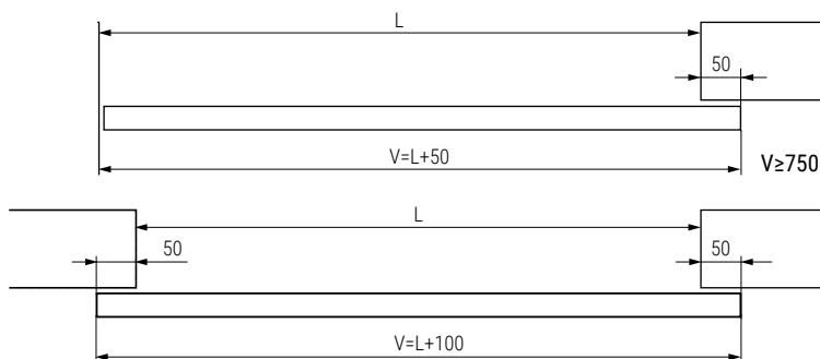
Aplicación con perfil al techo con pared Application with profile for ceiling with wall
