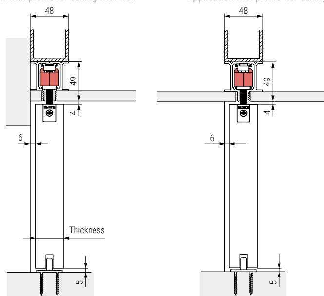
Aplicación con perfil al techo con pared Application with profile for ceiling with wall
