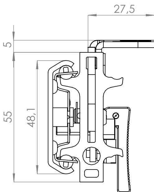
Vista Detalle 1:1
