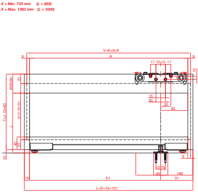
ACCESSORIES PLACEMENT (INTERMEDIATE POSITION) / POSIZIONAMENTO DEGLI ACCESSORI (POSIZIONE INTERMEDIA)
