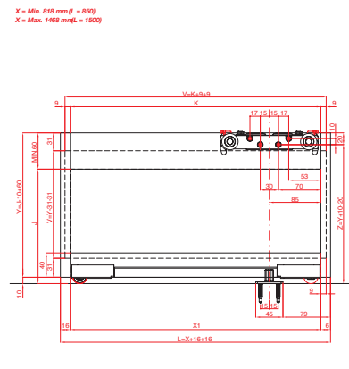
ACCESSORIES PLACEMENT (STANDARD POSITION) / POSIZIONAMENTO DEGLI ACCESSORI (POSIZIONE STANDARD)
