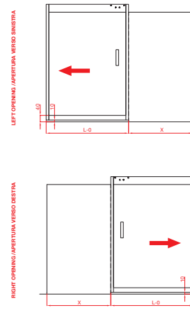
ACCESSORIES PLACEMENT (TOTAL OPENING POSITION) / POSIZIONAMENTO DEGLI ACCESSORI (POSIZIONE APERTURA TOTALE)
