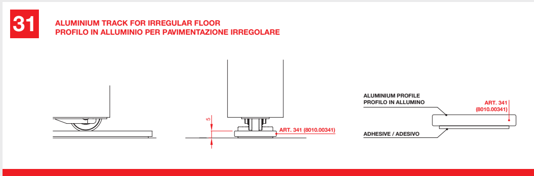
MEASUREMENTS DESCRIPTION / DESCRIZIONE MISURE
