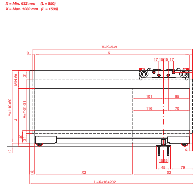
ACCESSORIES PLACEMENT (TOTAL OPENING POSITION) / POSIZIONAMENTO DEGLI ACCESSORI (POSIZIONE APERTURA TOTALE)
