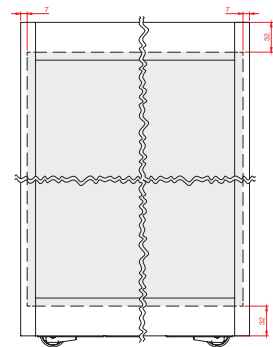
ACCESSORIES PLACEMENT (INTERMEDIATE POSITION) / POSIZIONAMENTO DEGLI ACCESSORI (POSIZIONE INTERMEDIA)
