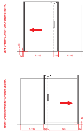
ACCESSORIES PLACEMENT (INTERMEDIATE POSITION) / POSIZIONAMENTO DEGLI ACCESSORI (POSIZIONE INTERMEDIA)
