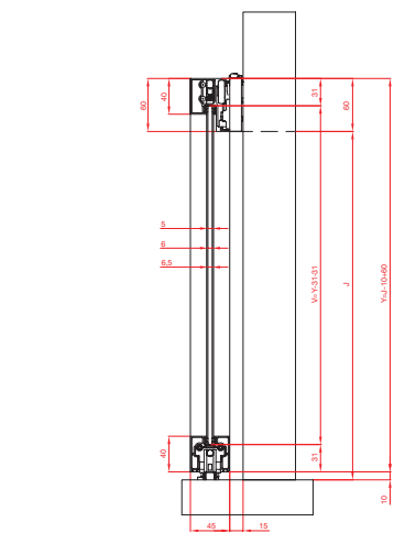
ACCESSORIES PLACEMENT (INTERMEDIATE POSITION) / POSIZIONAMENTO DEGLI ACCESSORI (POSIZIONE INTERMEDIA)
